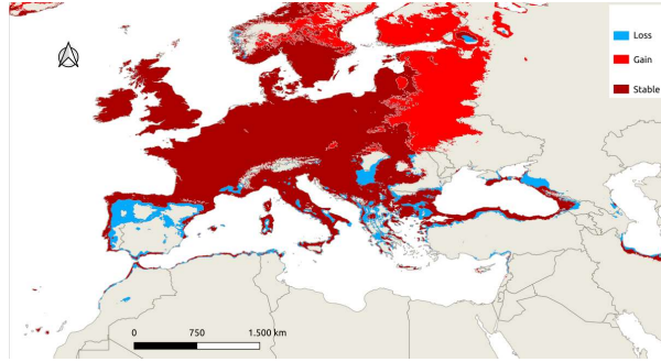
MPI-ESM1-2-HR SSP3-7.0
