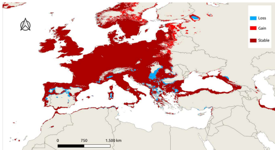
MPI-ESM1-2-HR SSP3-7.0
