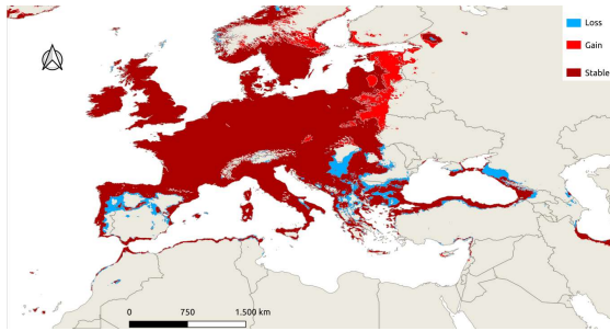
MPI-ESM1-2-HR SSP3-7.0
