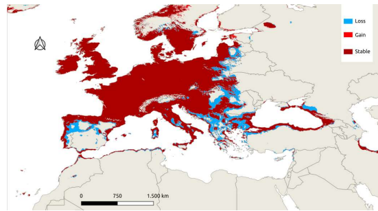
IPSL-CM6A-LR SSP5-8.5
