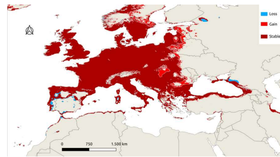
MPI-ESM1-2-HR SSP5-8.5
