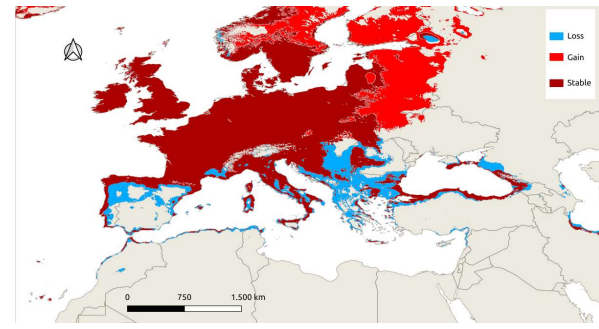
MPI-ESM1-2-HR SSP5-8.5
