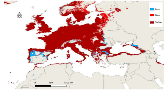
MPI-ESM1-2-HR SSP5-8.5
