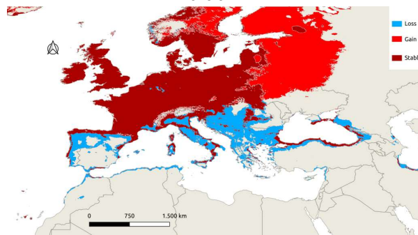
IPSL-CM6A-LR SSP5-8.5
