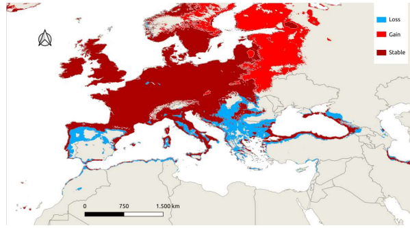
IPSL-CM6A-LR SSP5-8.5
