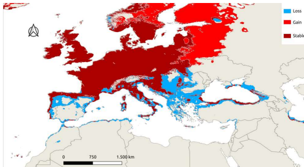
MPI-ESM1-2-HR SSP3-7.0
