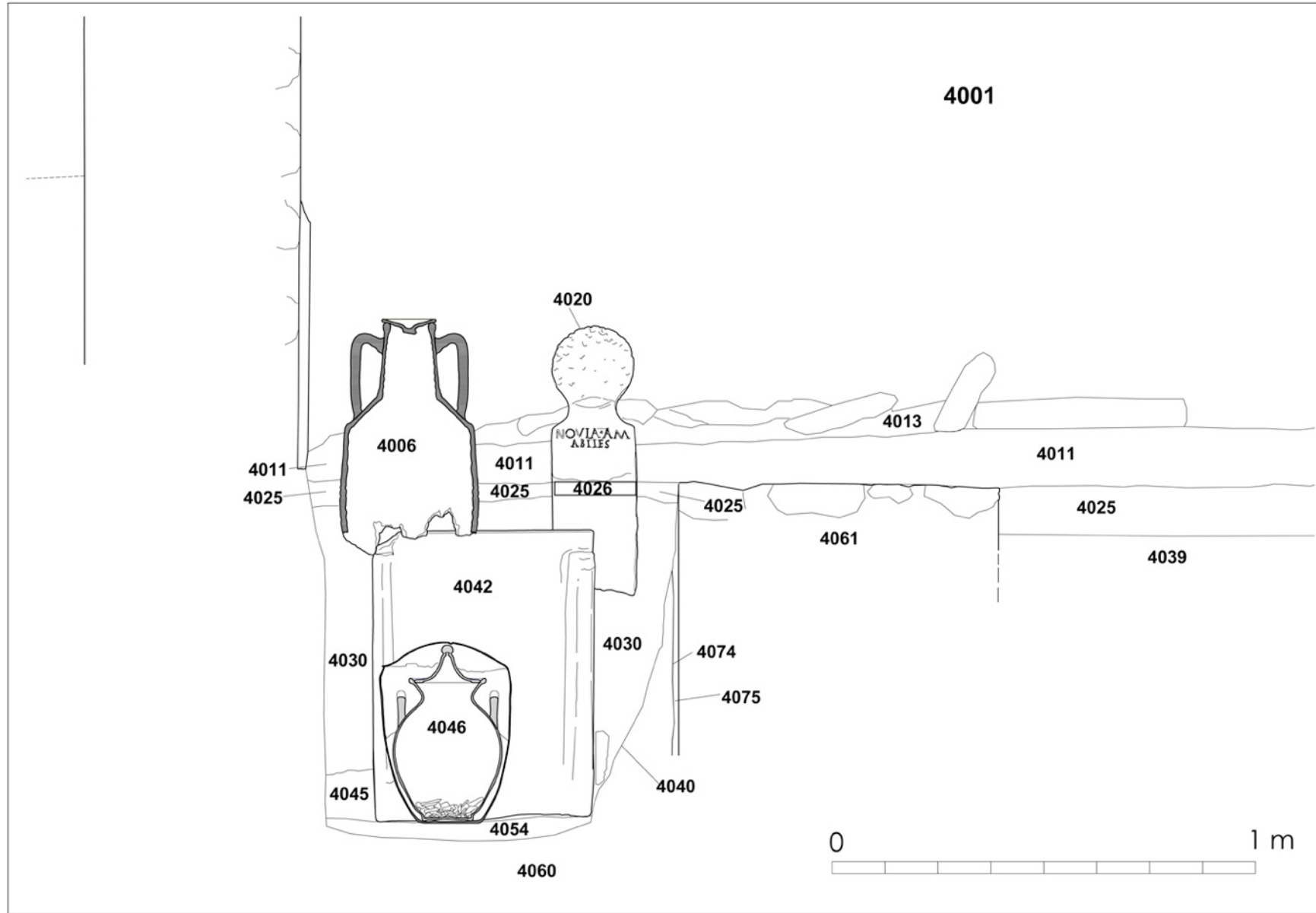
Suppl. Fig. 16. Detail of west-east section of the tomb of Marcus Venerius Secundio. (P. Mas. By permission of the Ministero per i Beni e le Attività Culturali e per il Turismo-Parco Archeologico di Pompei. Reproduction prohibited.)
