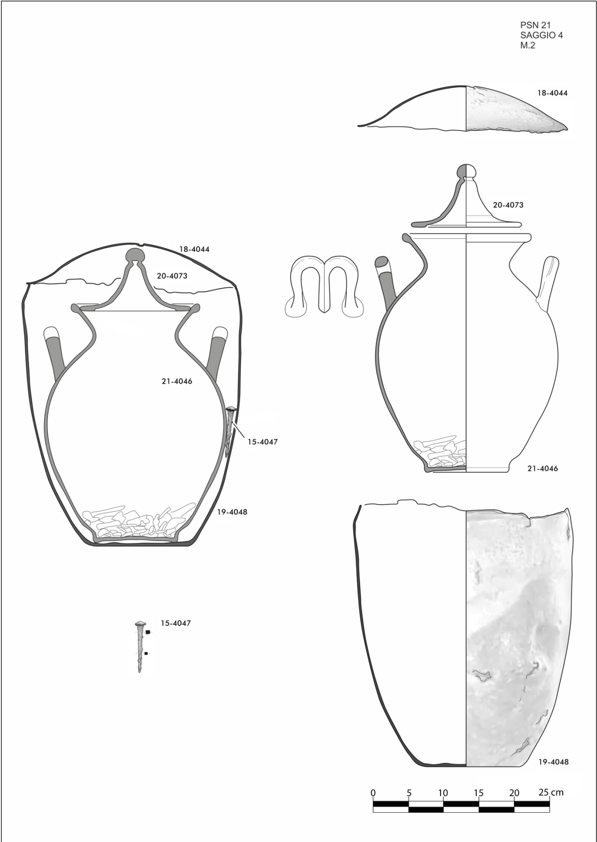
Suppl. Fig. 19. Detail drawings of the cinerary urn of Novia Amabiles and its metal container. (P. Mas. By permission of the Ministero per i Beni e le Attività Culturali e per il Turismo-Parco Archeologico di Pompei. Reproduction prohibited.)
